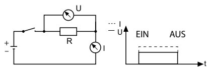
Strom-/Spannungsverlauf beim Schalten einer Relaisspule Abb.2
